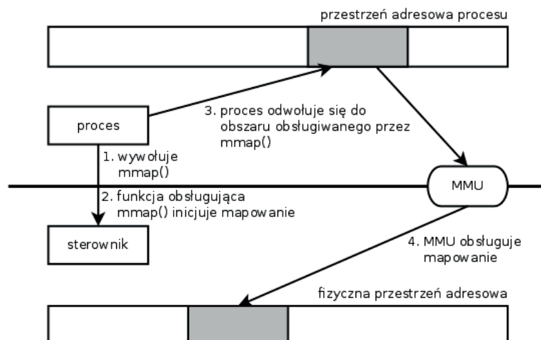
Ilustracja 1: schemat mmap
